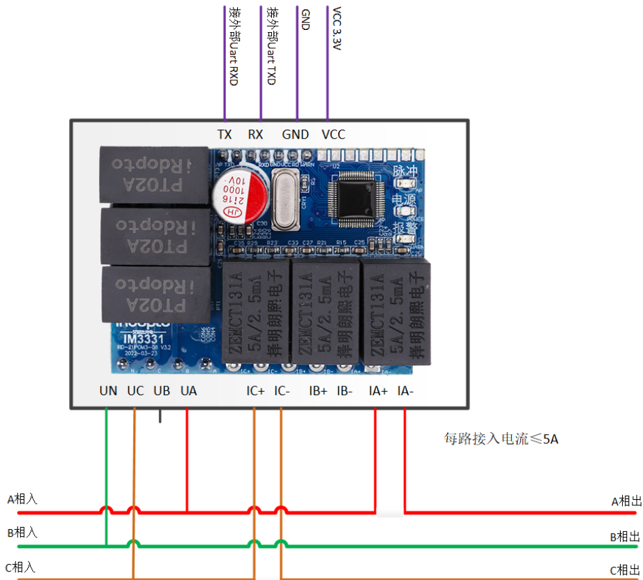
IM3331三相三线板载CT接线示意图
