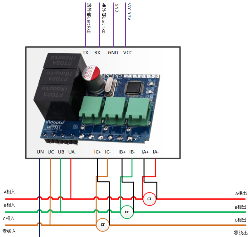
IM3331三相四线外置CT接线示意图
