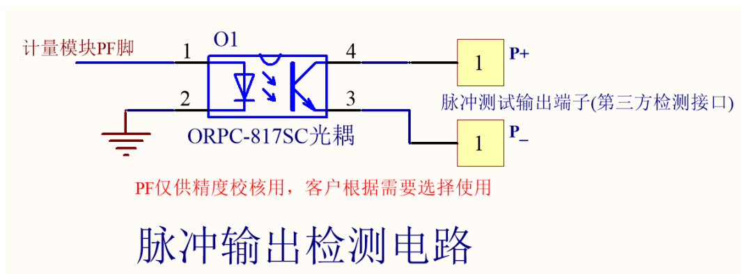
IM1281V 脉冲检测接口接线示意图
